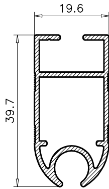
10.229 PESO TCO: 0.473 PERIMETRO: 0.27
