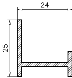
1.373 PESO TCO: 0.276 PERIMETRO: 0.12
