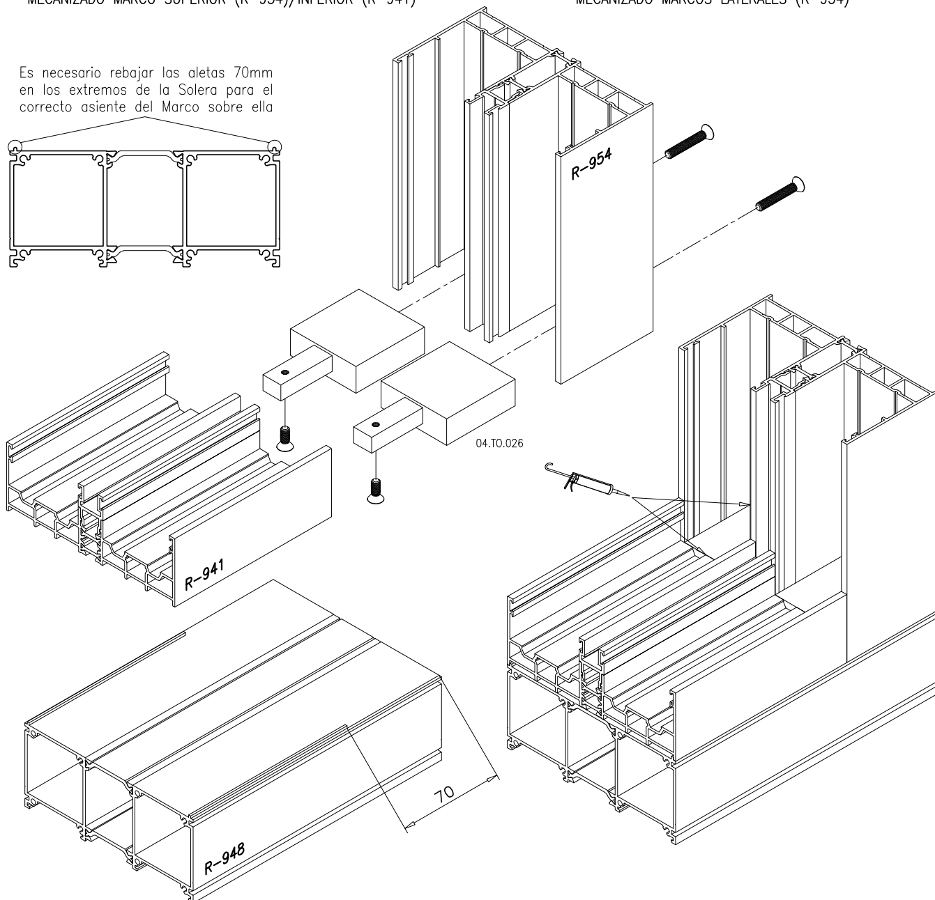
MECANIZADO MARCO SUPERIOR (R-954)/INFERIOR (R-941)
