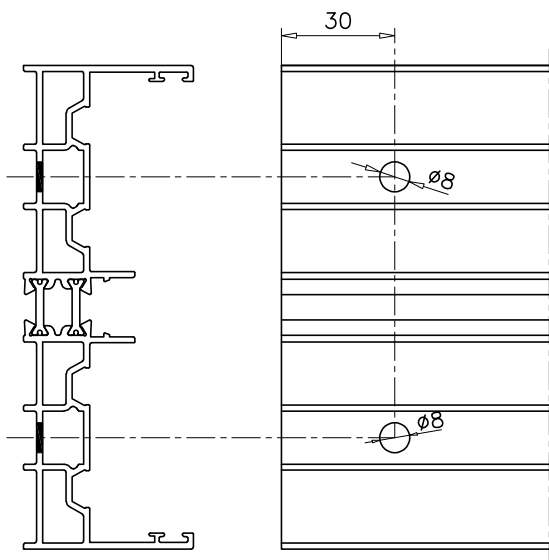
MECANIZADO MARCO SUPERIOR (R-954)/INFERIOR (R-941)
