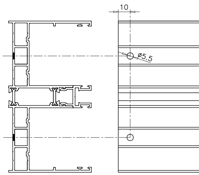
MECANIZADO MARCOS LATERALES (R-954)
