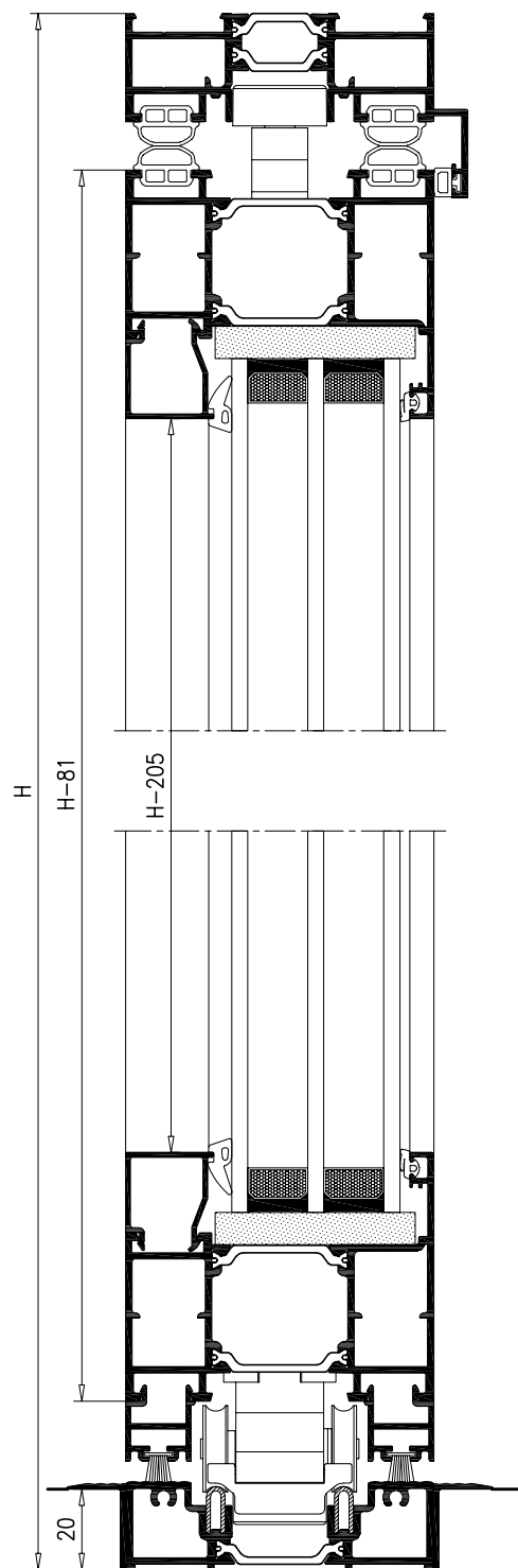
MARCO INFERIOR EMBUTIDO CON O SIN DRENAJE OCULTO
