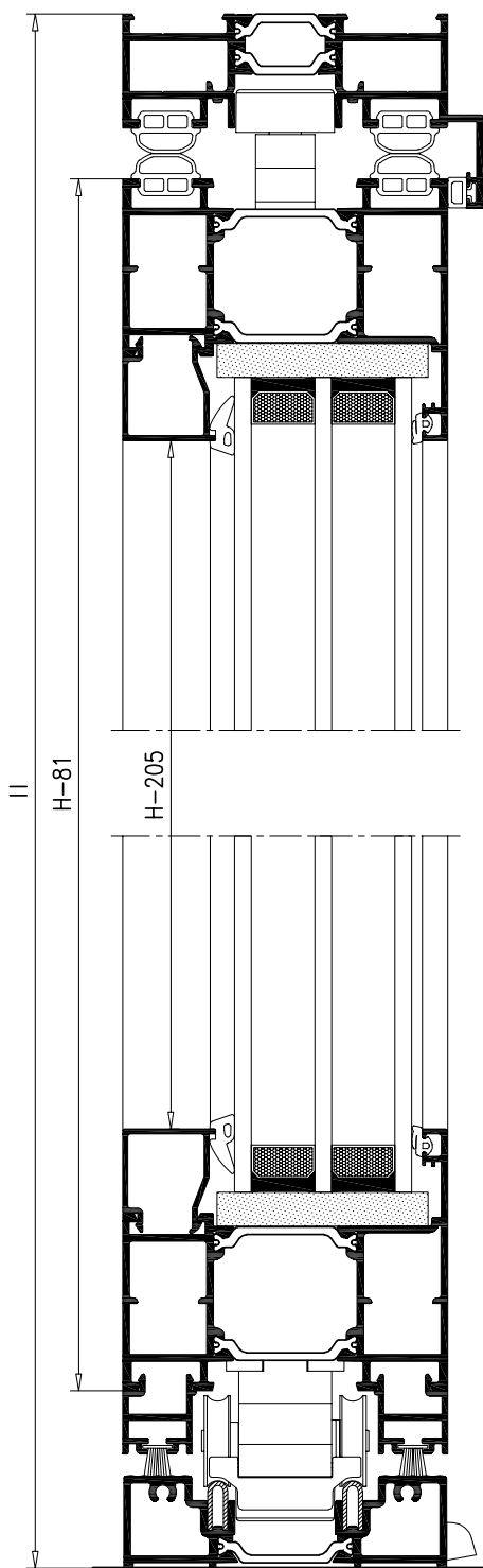
MARCO INFERIOR SUPERPUESTO
