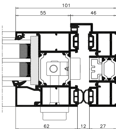
SECCIÓN E-160
