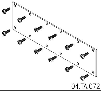
Tapa para Solera R-949
