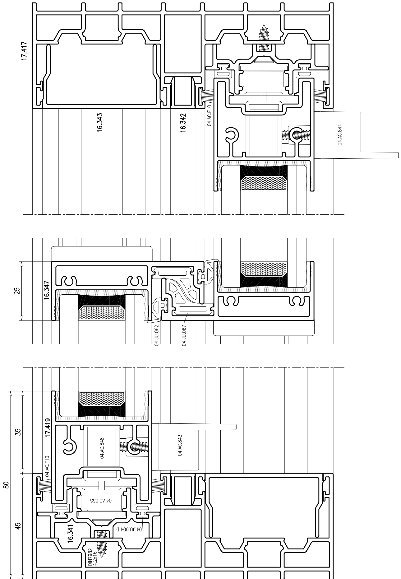
SECCION HORIZONTAL 2 HOJAS
