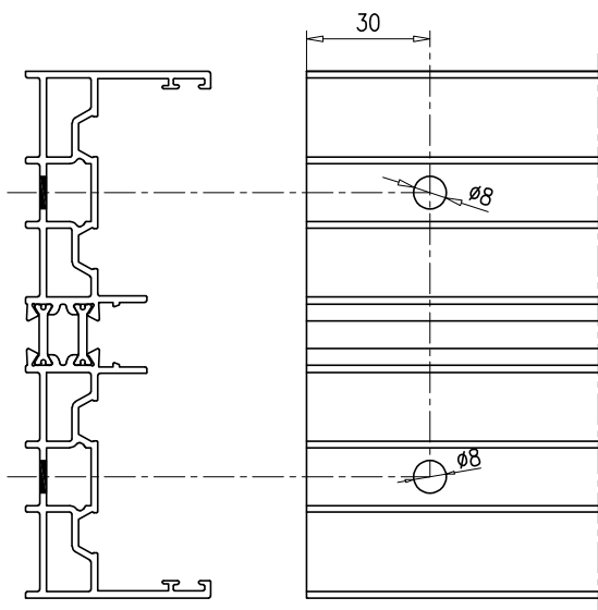
MECANIZADO MARCO SUPERIOR/INFERIOR
