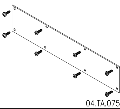
Tapa para Solera R-953
