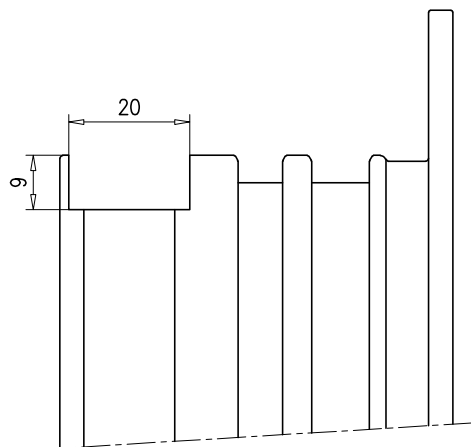
Mecanizado "B"
