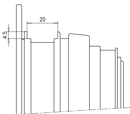
Mecanizado "A"
