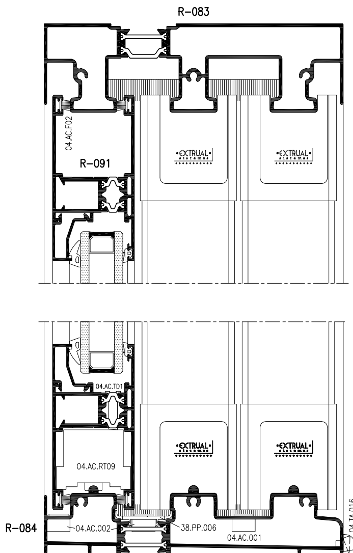
SECCION B-B'
