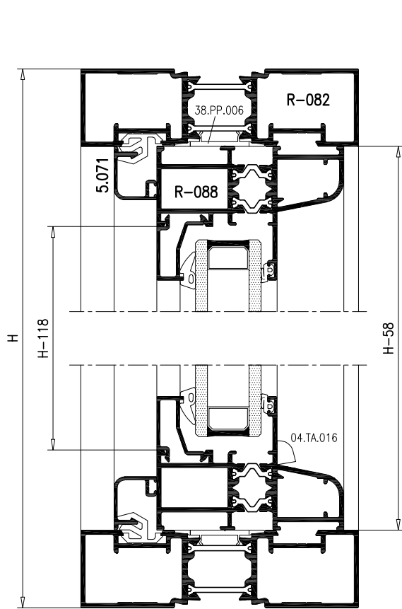
SECCION A-A'
