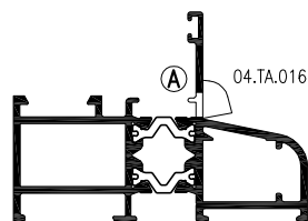
MARCO FIJO
