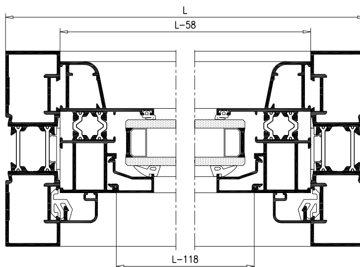
SECCION B-B'
