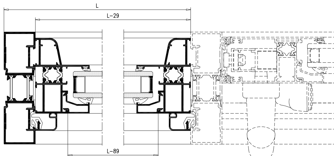
SECCION B-B'
