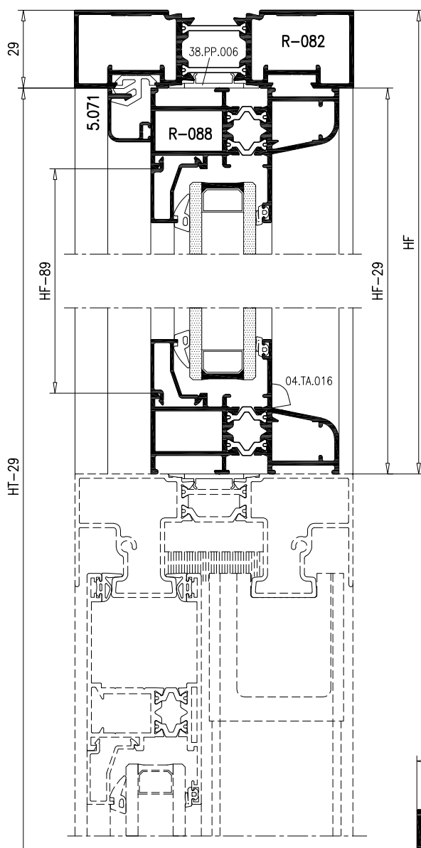
SECCION A-A'
