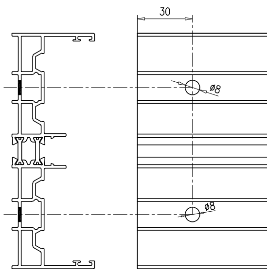
MECANIZADO MARCO SUPERIOR/INFERIOR
