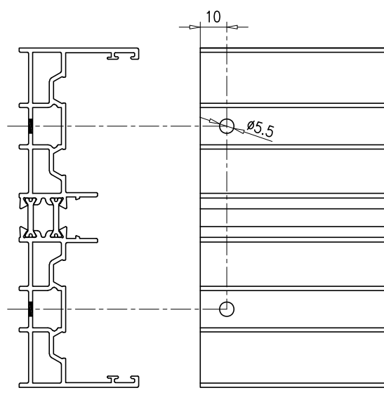
MECANIZADO MARCOS LATERALES
