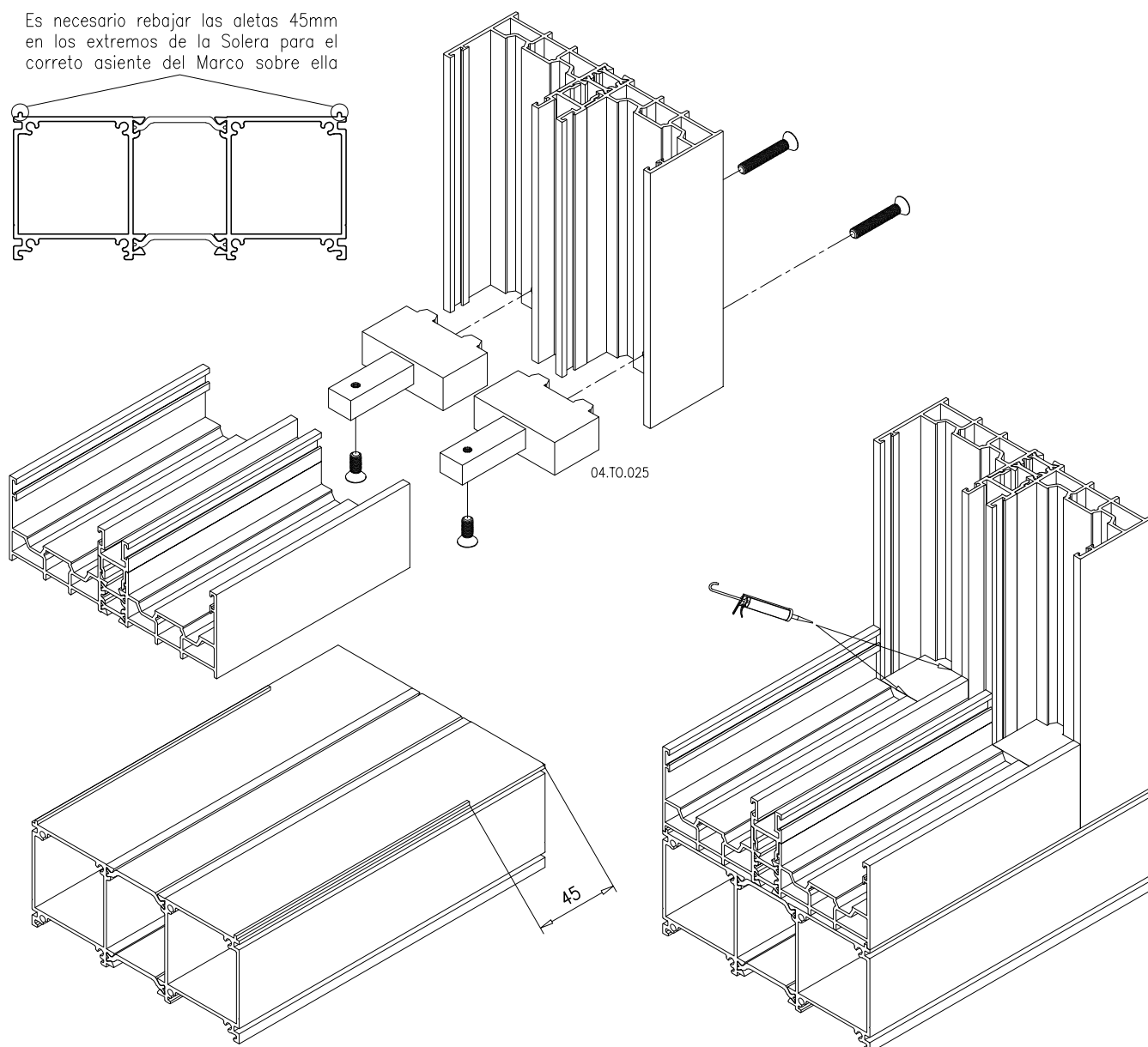
MECANIZADO MARCO SUPERIOR/INFERIOR
