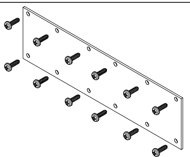
Tapa para Solera R-949
